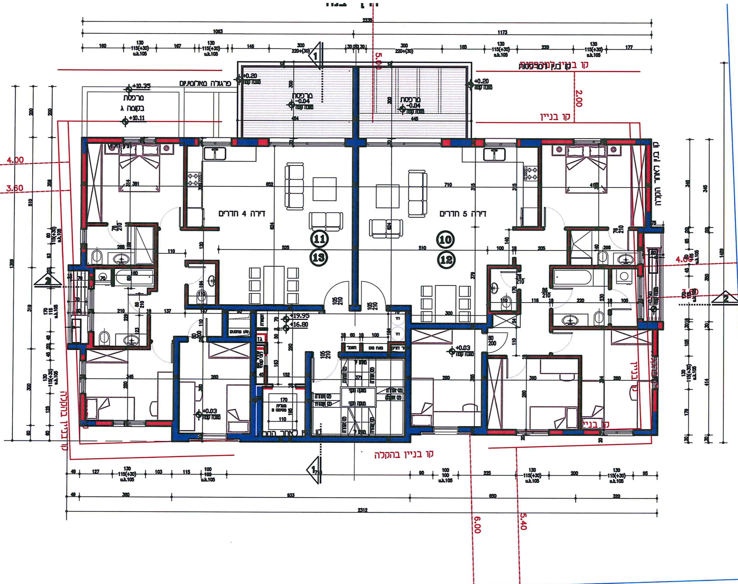
קומה 6,5 קנ"מ 1:100
