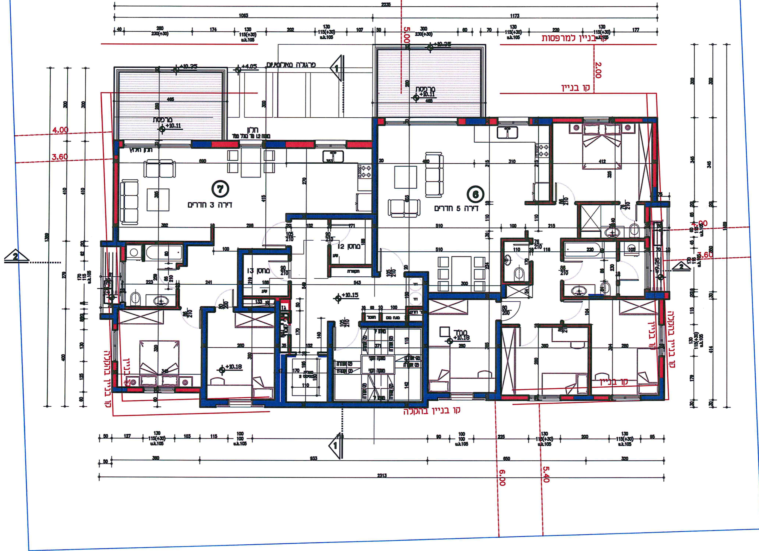
קומה 3 קנ"מ 1:100
